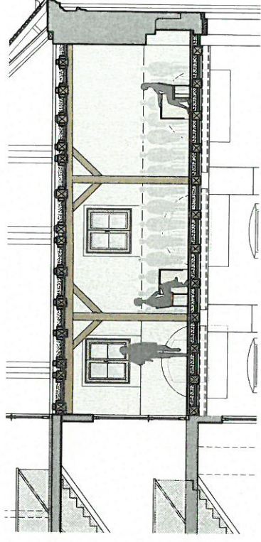
SCHNITT C-C
